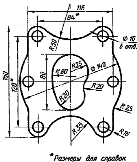
Чертеж 2
